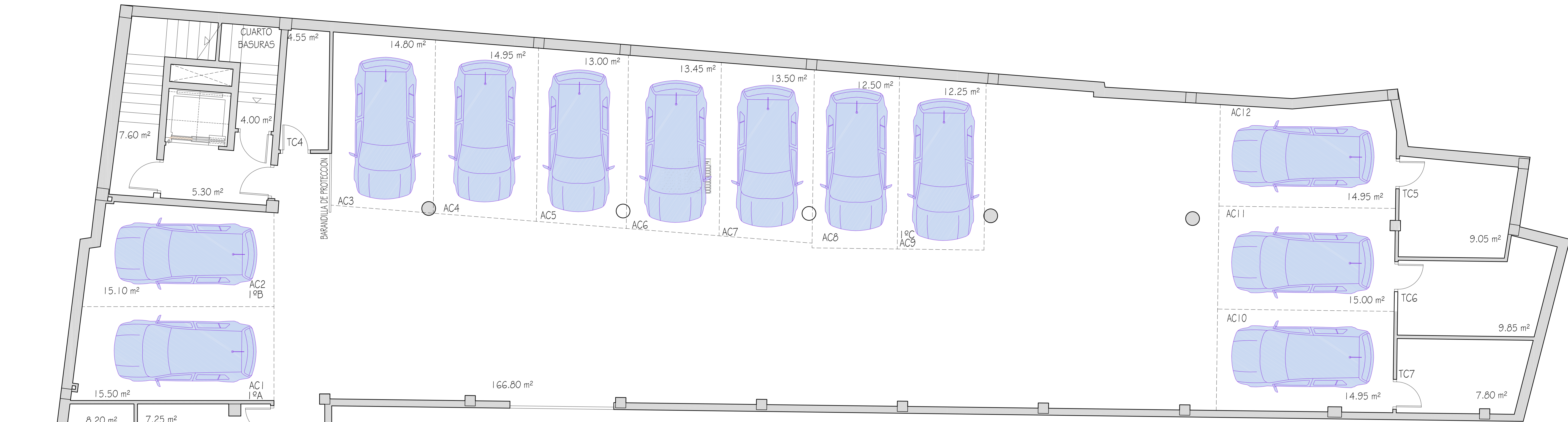
PLANTA SOTANO
